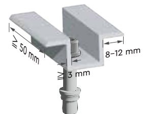
Abmessungen der Klemmen
