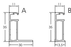
Rahmenquerschnitt
