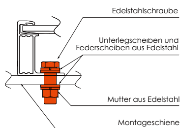
Schraubmontage der Module
