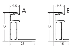
Rahmenquerschnitt
